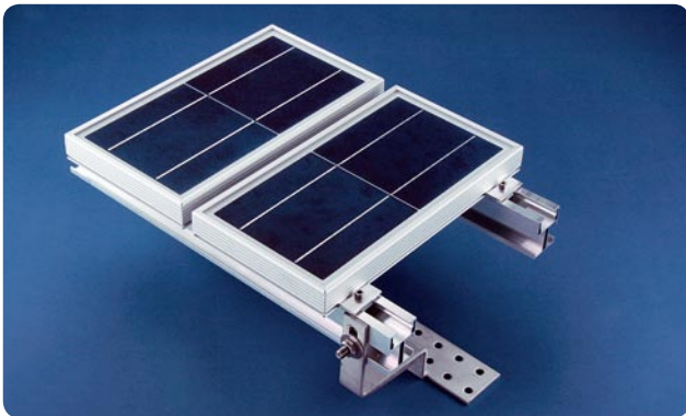
Das patentierte Profilink-System: die flexible Lösung für die Schrägdachmontage von gerahmten und ungerahmten Modulen.
