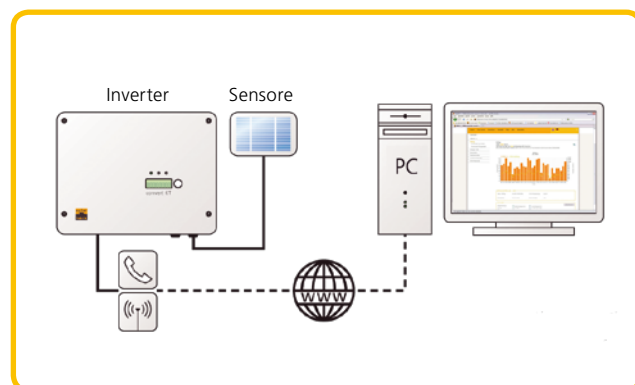
L'inverter del vostro impianto fotovoltaico invia i rendimenti al server.
