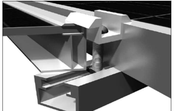
Beispiel 1 – Klemmflügel
